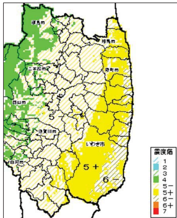
【福島県沖地震の震度分布図】
