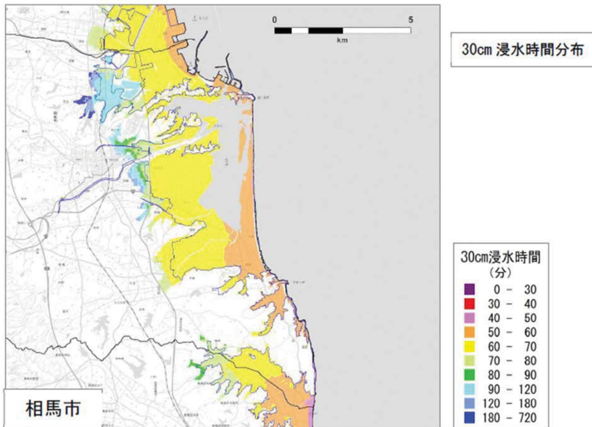
(7) 想定東北地方太平洋沖地震津波による 30 c m浸水時間分布
