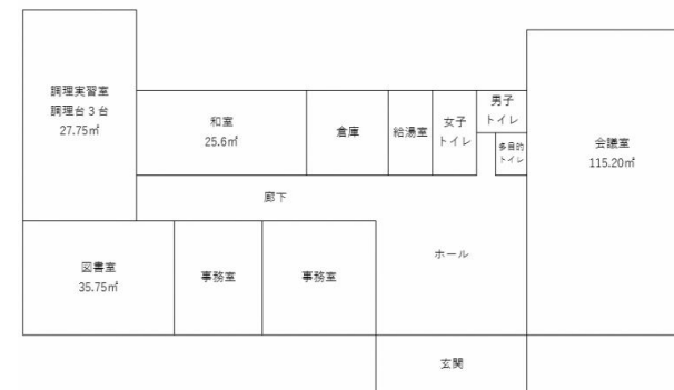
山上公民館 配置図
